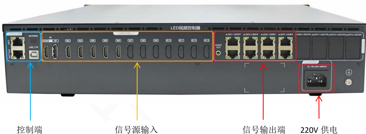
后面板
